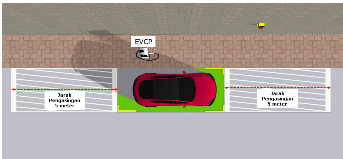
Rajah 8: EVCP Jenis Peranti DC di Dalam Bangunan Dengan Keluasan Lantai Kurang 216 m 2 Hendaklah Dipisahkan Dengan Jarak Pengasingan 5 m Daripada TLK Bukan EV
