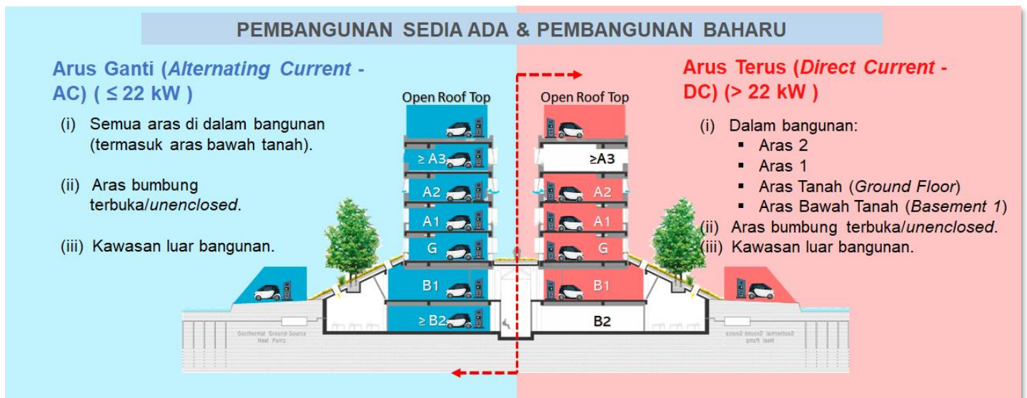
Rajah 3: Penyediaan EVCB Mengikut Jenis Peranti Pengecasan dan Lokasi
