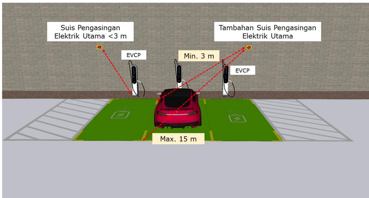
Rajah 12: Keperluan Tambahan Suis Pengasingan Elektrik Utama
